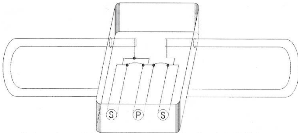
S - transformační a symetrizační smyčka ( \lambda/2 \cdot k ) P - přívod
