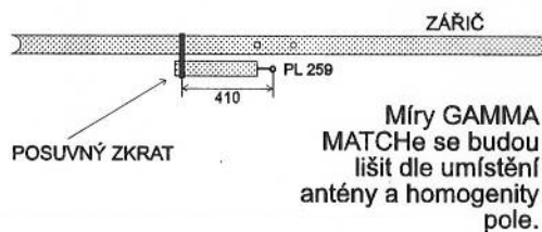
DETAIL PŘÍZPŮSOBNÍ A TRANSFORMACE (GAMMA MATCH)
