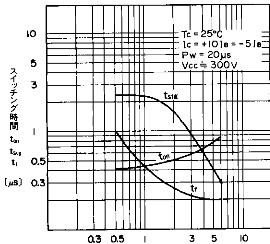
コレクタ電流 I_c (A) スイッチング時間—コレクタ電流特性 Switching Time
