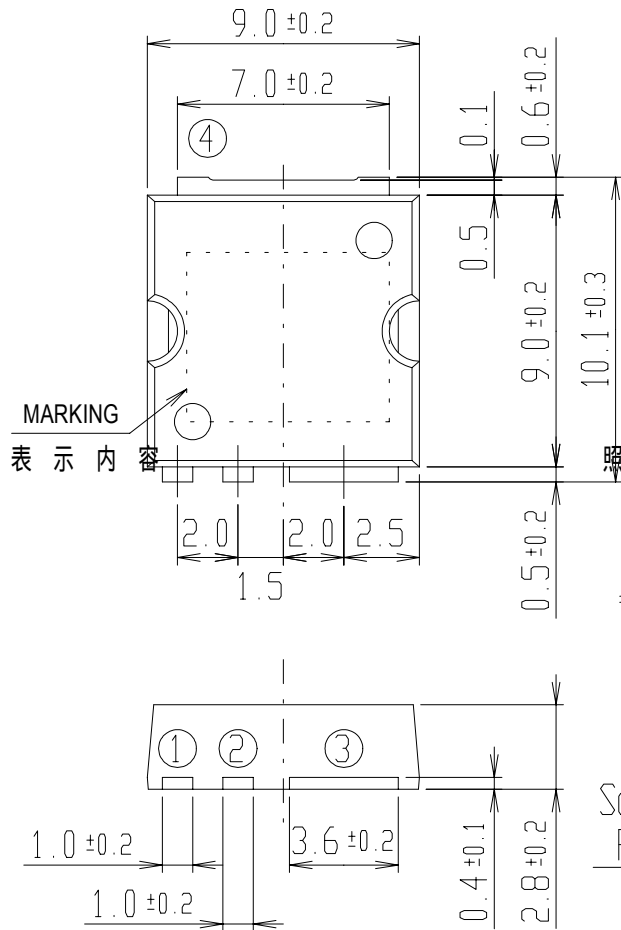
Fig. 1 P 矢視図
