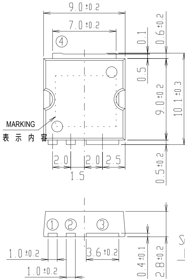
Fig. 1 P 矢视图
