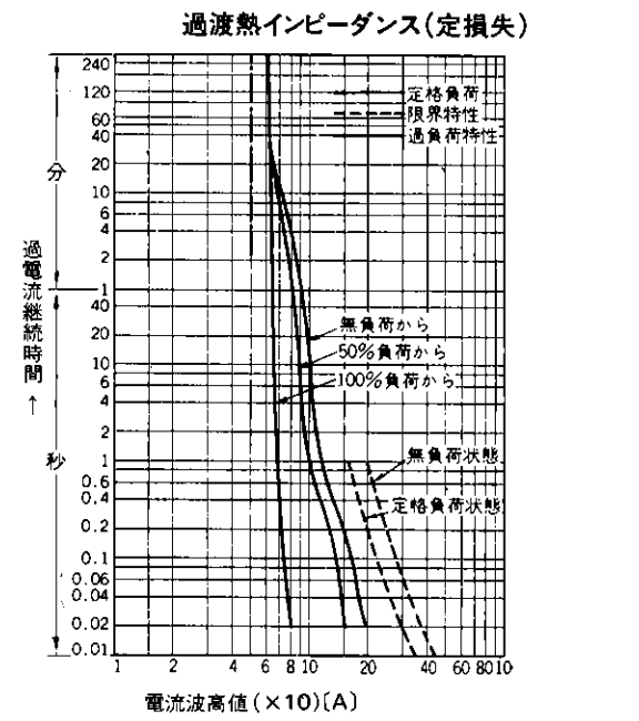
過負荷電流—時間 (冷却体AG01-6B) 自冷 50Hz正弦波電流 (通流角180°)
