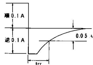
注1 逆回復時間測定波形
