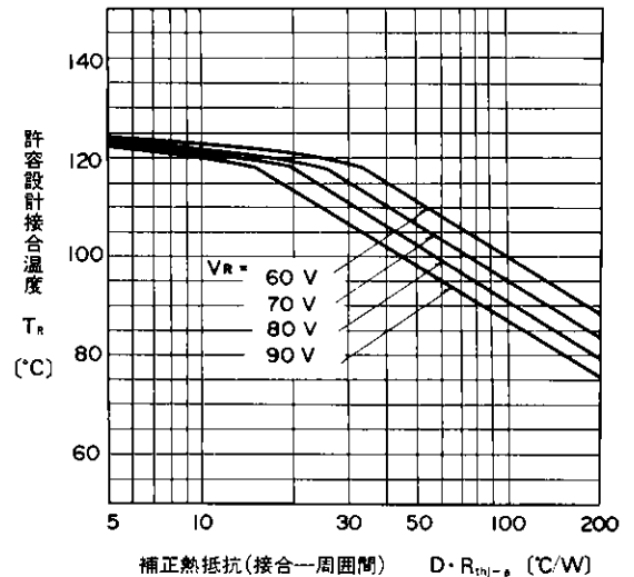
許容設計接合温度特性 T_R \cdot D \cdot R_{thj-a} Characteristics
